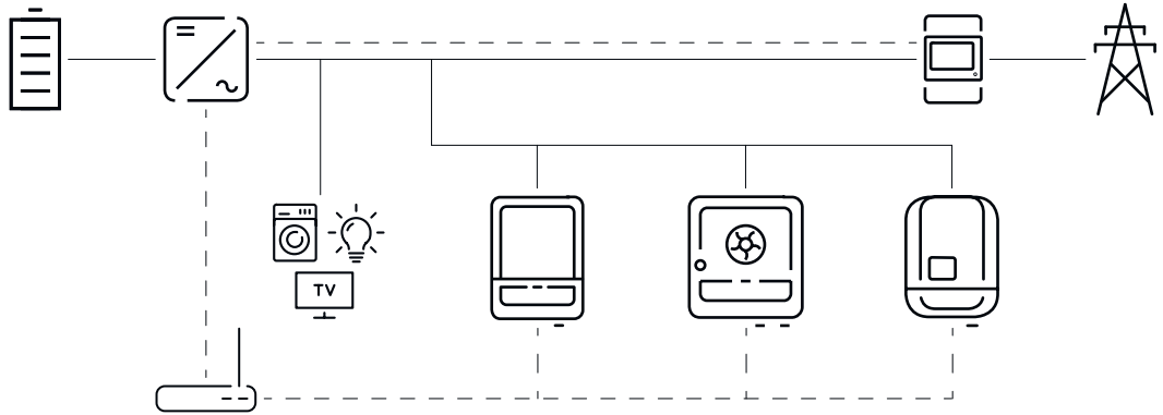
Exemple de schéma de connexion de la limite d'injection dynamique avec plusieurs onduleurs
