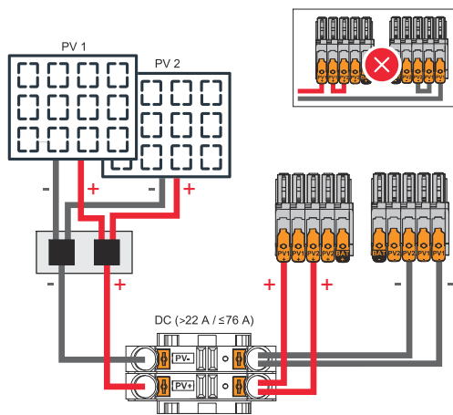
Chaînes de modules solaires combinées avec un courant total supérieur à 22 A ( I_{dcmax} ).
