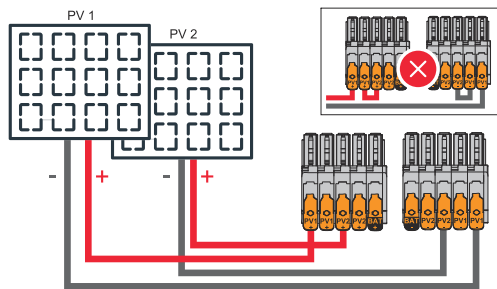
PV 1 inférieur ou égal à 44 A ( I_{SC\ PV1} ) PV 2 inférieur ou égal à 32 A ( I_{SC\ PV2} )
