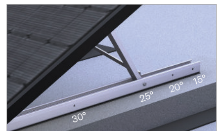
Triángulos para cuatro ángulos de elevación
