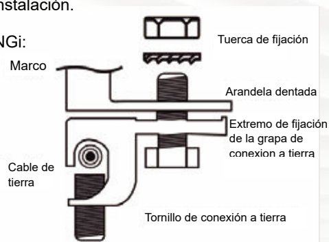
Figura 10 Conexión a tierra de un módulo a través de un tornillo
