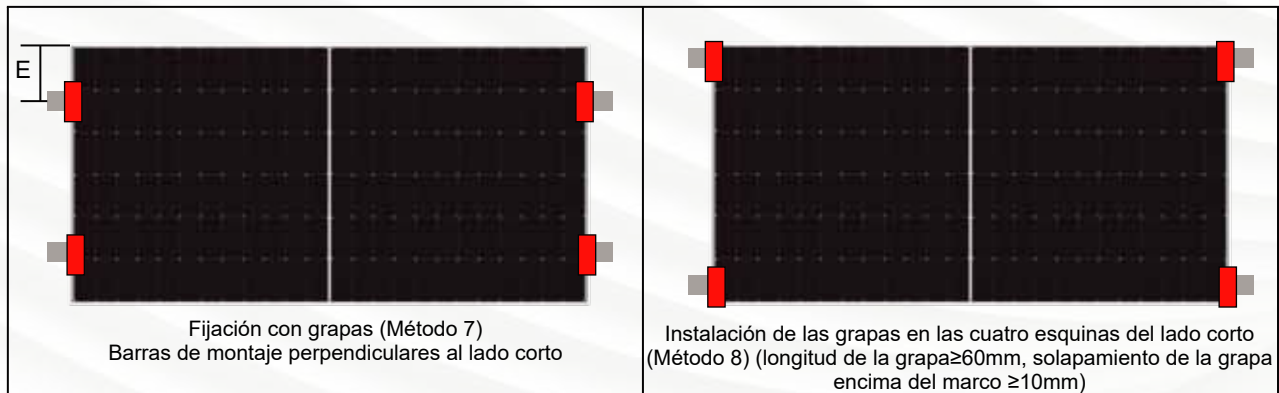
Figura 8 Diagrama de la posición de instalación de un módulo bifacial
