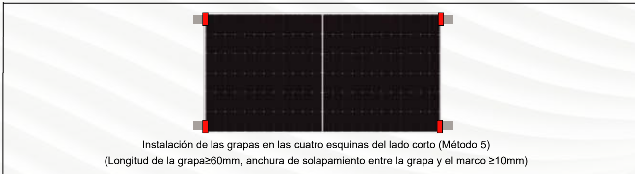
Figura 7 Diagrama de la posición de instalación del módulo mono facial
