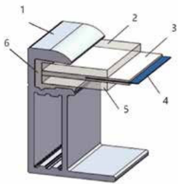
Módulos de doble acristamiento (con marco)
