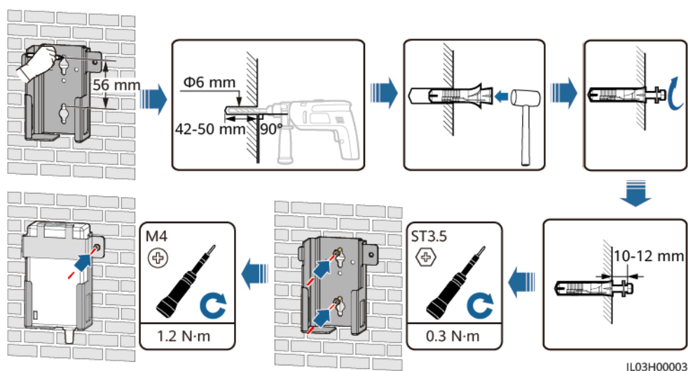
Figura 3-9 Instalación sobre pared (modo 1)
