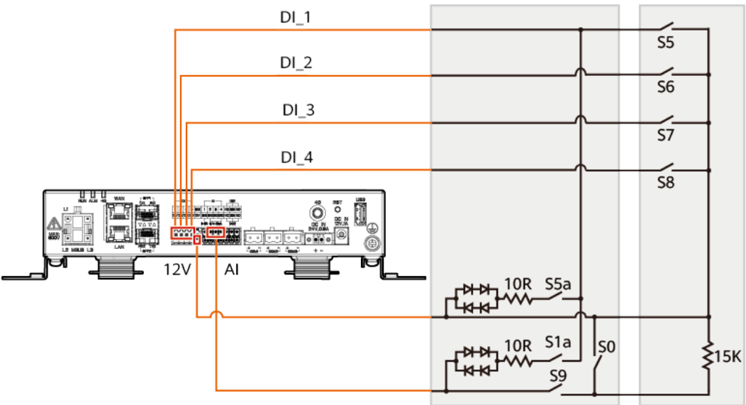
Figura 6-79 Diagrama eléctrico para la función DRM
